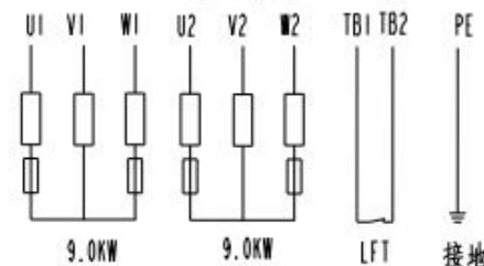
电加热接线图
